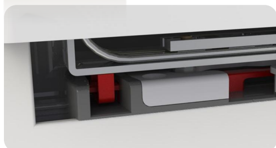
secuLock 500 verbindet Flügel und Blendrahmen.
